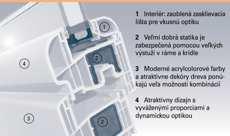
Detail štlupu
